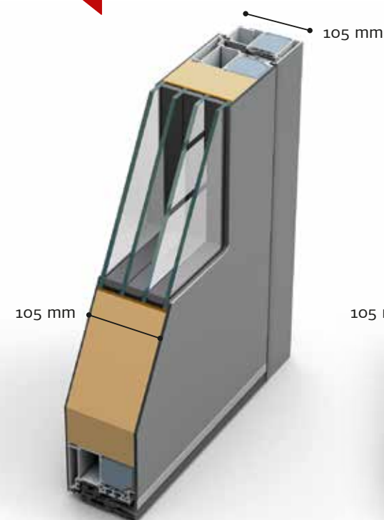
PROFIL ADS 105
