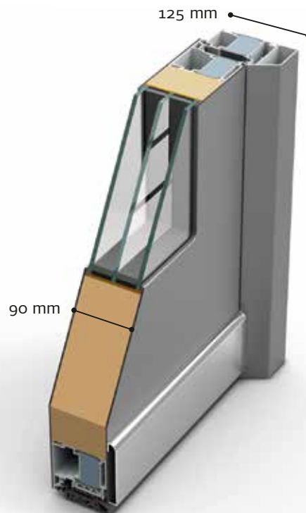
PROFIL ADS 125
