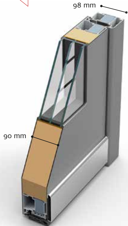
PROFIL ADS 95
