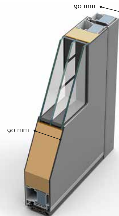
PROFIL ADS 90
