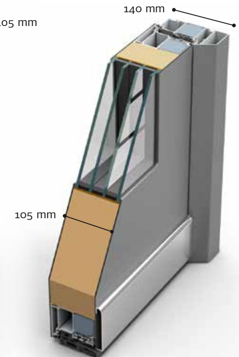
PROFIL ADS 140
